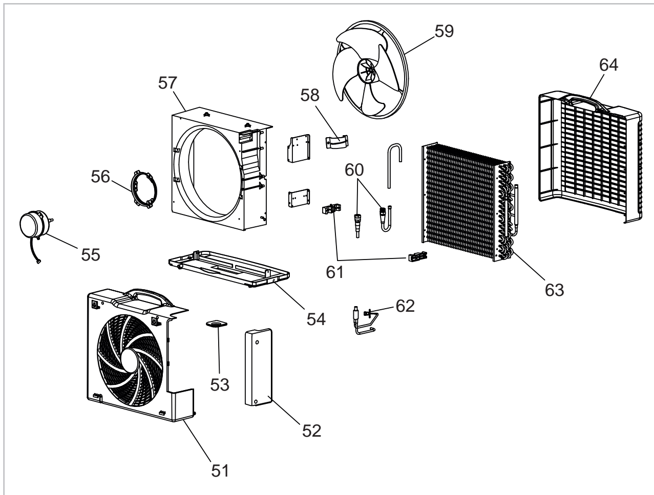
Abb. 20: Explosionszeichnung Außenteil
