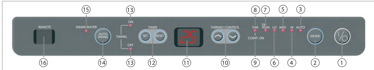
Abb. 3: Bedienungstableau
