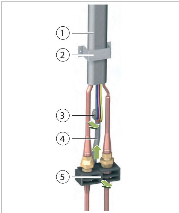
Abb. 13: Demontage Verbindungsleitung
